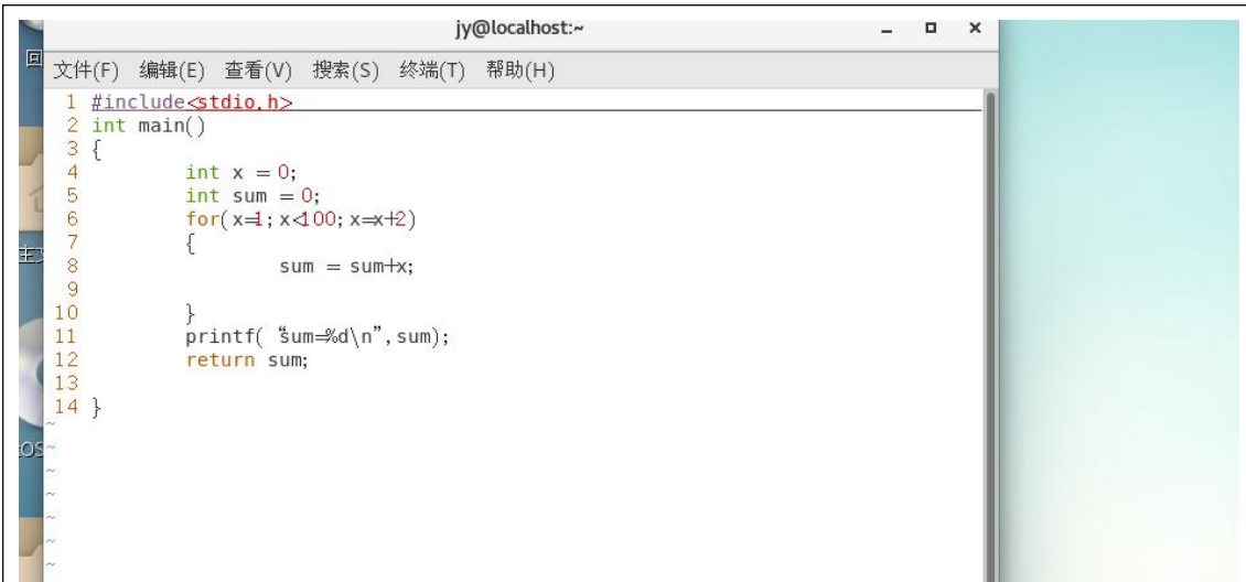
图 19 vim 编写了一个 C 语言程序
