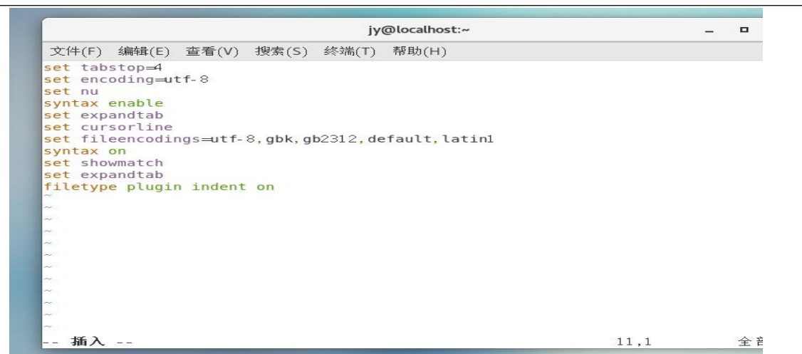
图 32 在.vimrc 文件中填写需要的配置
